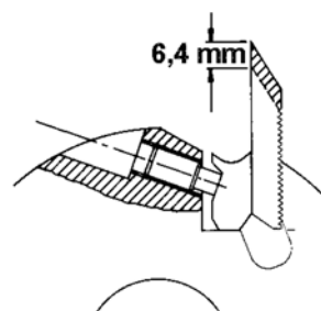
Stellung des Messers vorgestellt (max. 6,4 mm = 4 Zähne)
